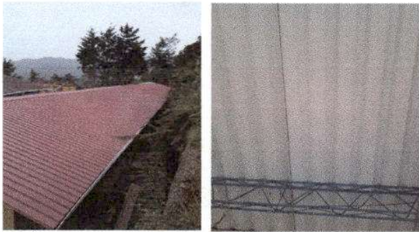
Foto 1: Módulo 2, Sustitución de lámina por lámina troquelada, sustitución de capote y sustitución de elementos de fijación.
